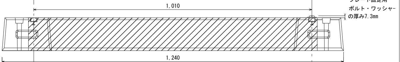
アルミレール内側設置 最大アンカーピッチ
