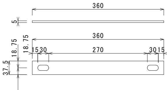
連結金具 詳細図
