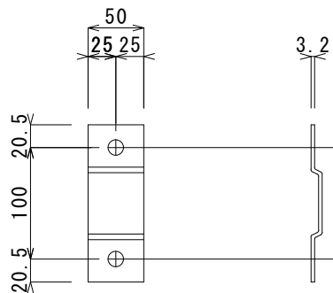
連結金具 詳細図
